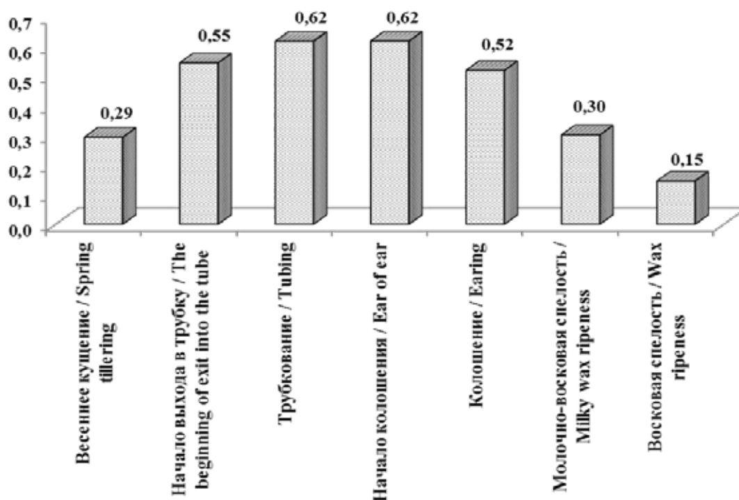
Рис. 1. Коэффициенты корреляции между NDVI и урожайность озимой пшеницы, в среднем за 2015–2017 гг. (значимость коэффициентов корреляции: p = 0,05–0,23 ; p = 0,01–0,30 )
