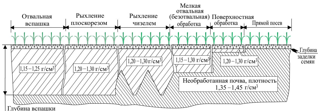
Рис. 2. Схема вертикального разреза обработанного слоя почвы при различных способах обработки. Представленные на рисунке величины плотности при различной обработке характерны для дерново-подзолистой почвы. На других типах почвы эти величины будут иными. И в данном случае они служат лишь для иллюстрации факта повышения плотности обработанных слоев в результате последовательного перехода от более интенсивной обработке к менее интенсивной.
